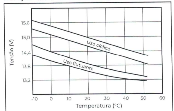
Relação entre tensão de carga e temperatura
